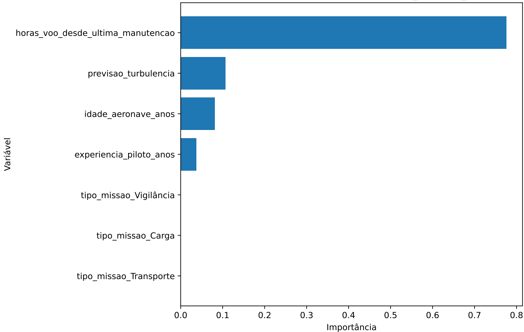
Top variáveis mais importantes — gradient_boosting_fallback
